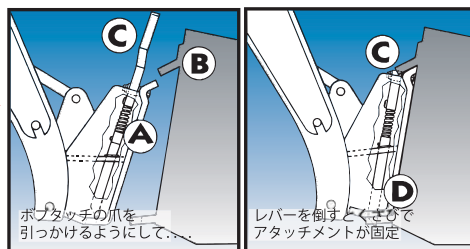
(側面図)
